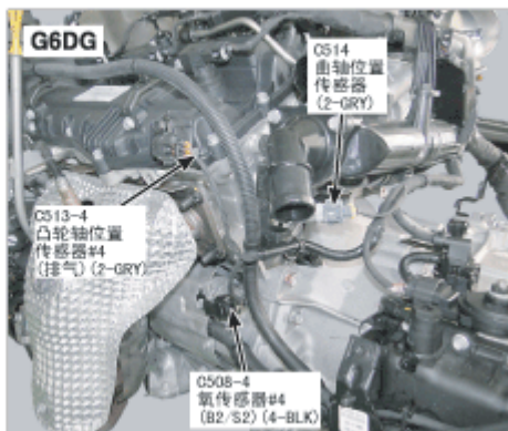
216. 发动机前左
