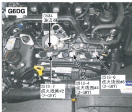
213. 发动机顶部
