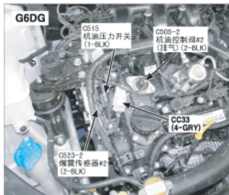
212. 发动机前右
