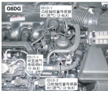
214. 发动机顶部
