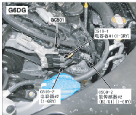
211. 发动机前右
